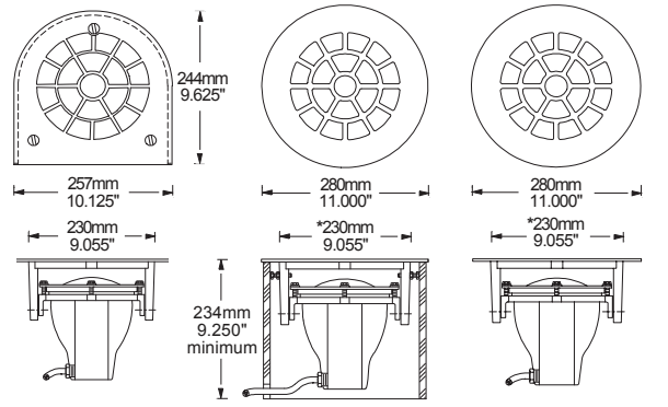
E150A + B57 B57 Slab Hanger E150A + B56-1 B56 on Pipe Stand (10" PVC Pipe, by others) E150A + B56 B56 Slab Hanger
